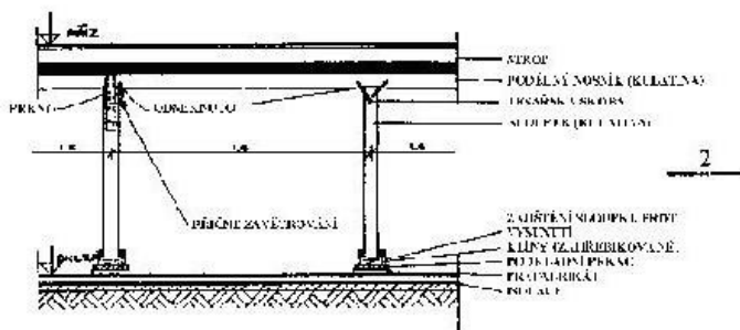
Pozdĺžny rez 2-2
